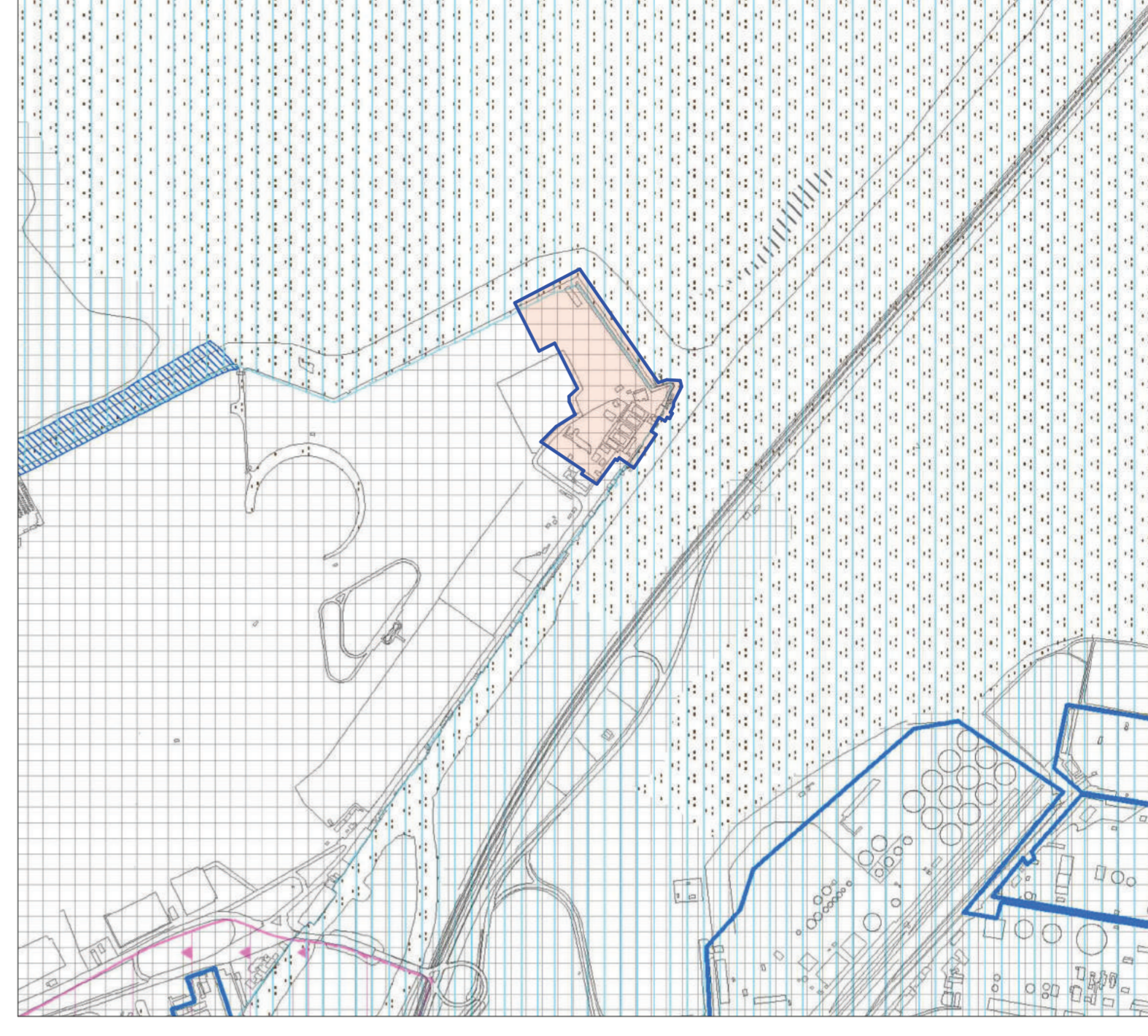
PAT - CARTA DELLA FRAGILITÀ | SCALA 1:10000
