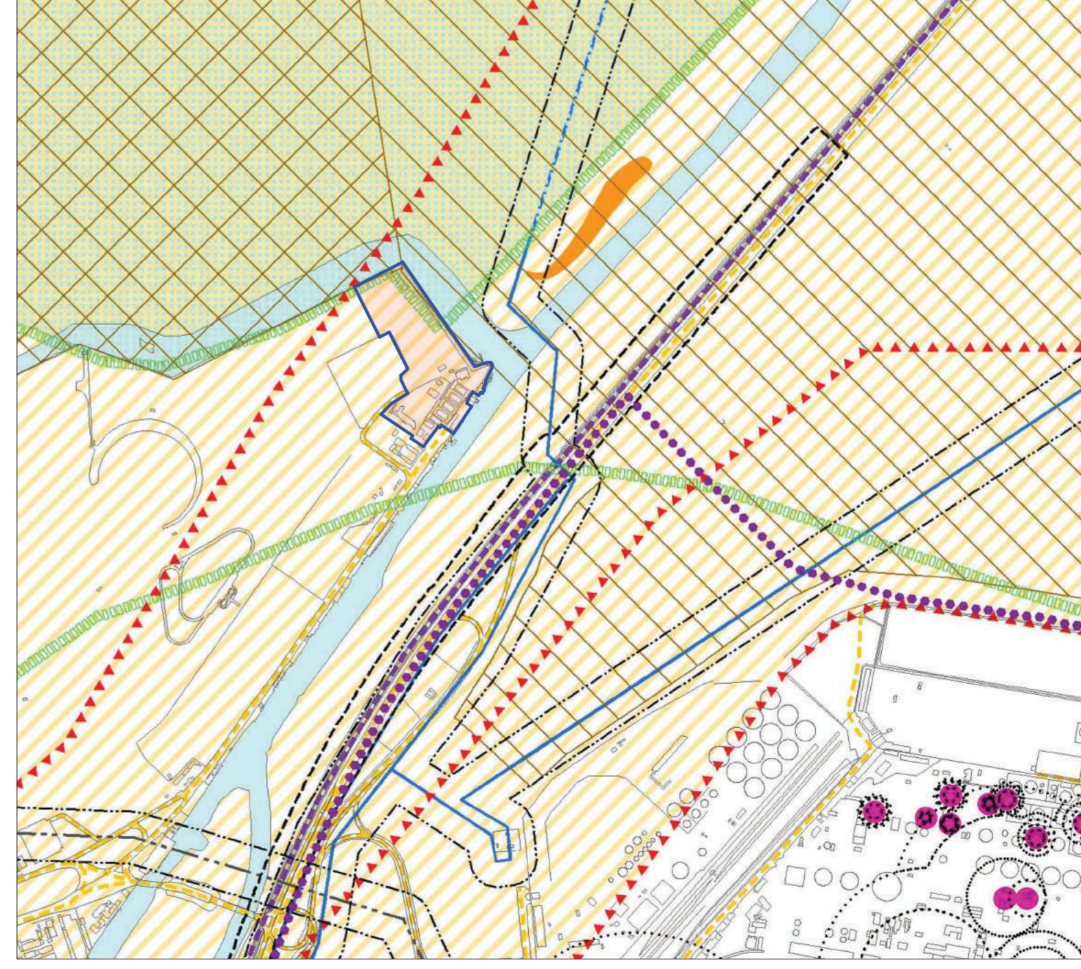
PAT - CARTA DEI VINCOLI | SCALA 1:10000
